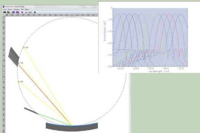
Echelle: Rowland design
